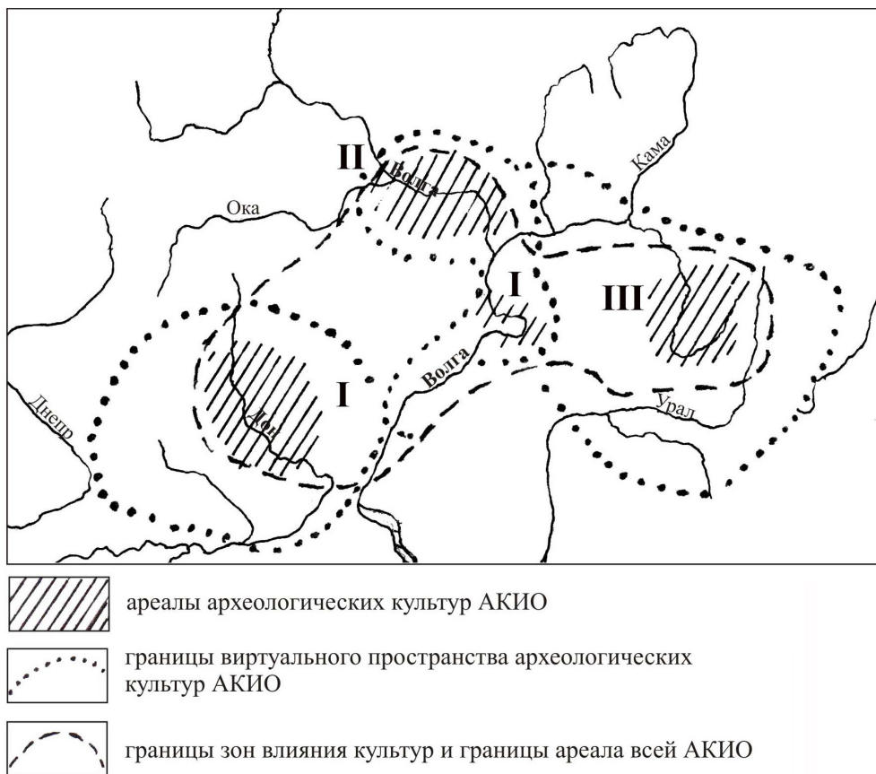
Рис. 1. Культурное пространство абашевской культурно-исторической общности (АКИО). I – доно-волжская абашевская культура; II – средневолжская абашевская культура; III – уральская абашевская культура Fig. 1. Cultural space of the Abashevo cultural and historical communion (ACHC). I – Don-Volga Abashevo culture; II – Mid-Volga Abashevo culture; III – Ural Abashevo culture
